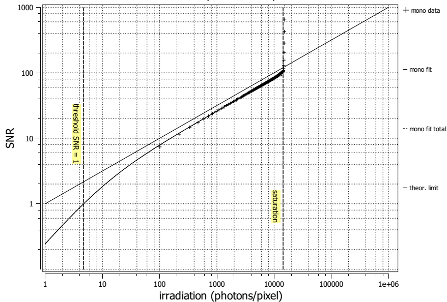
SNR mACC300142, 533 nm, 16.05.2023
